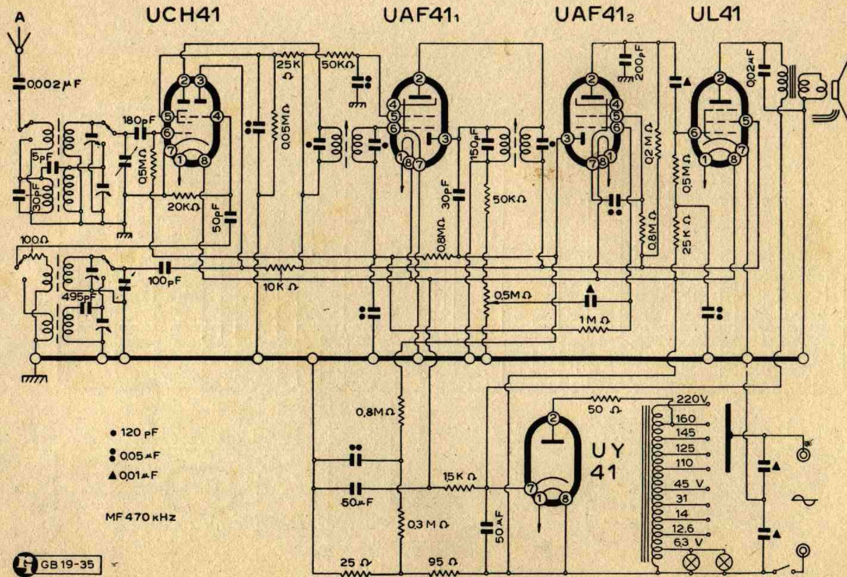
Lo schema elettrico del Mod. 485/1
